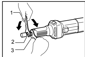
1. Llave 13 2. Tuerca 3. Llave 13
