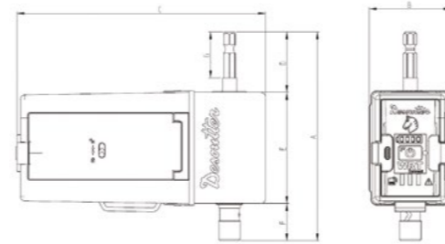
WRT4-Hex1/4, WRT10-Hex1/4, WRT20-Hex1/4
